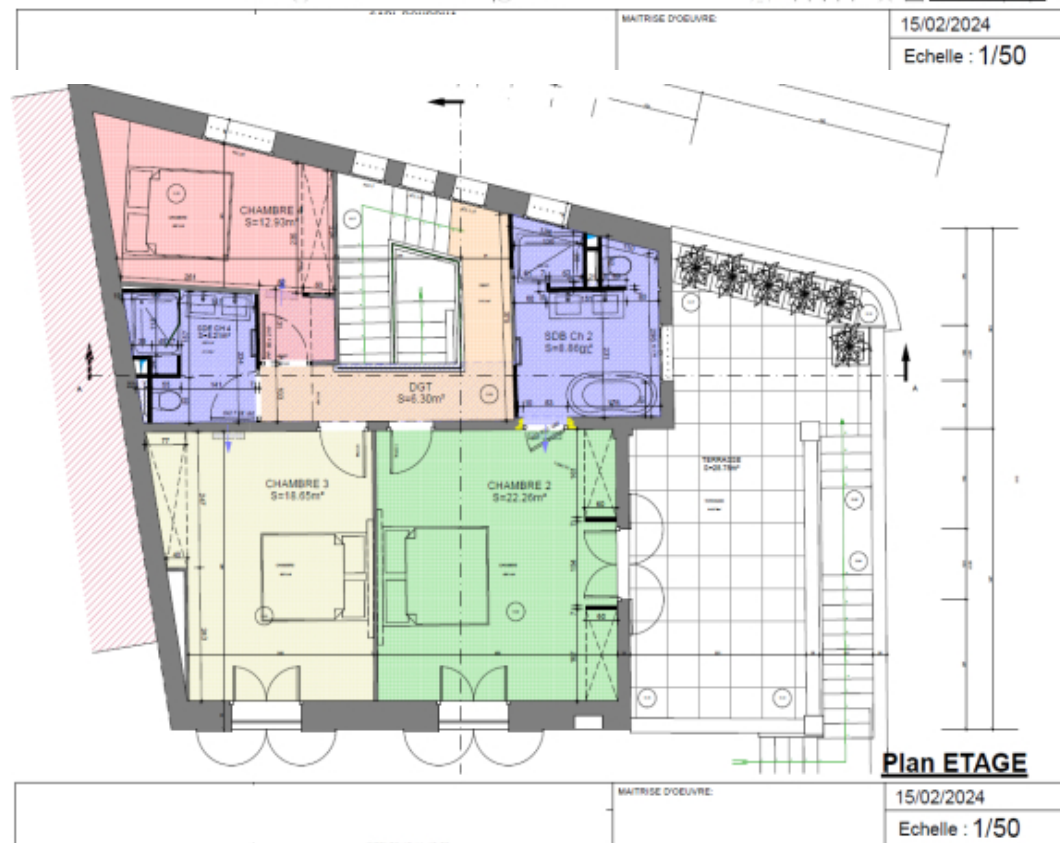
Plan RDC
